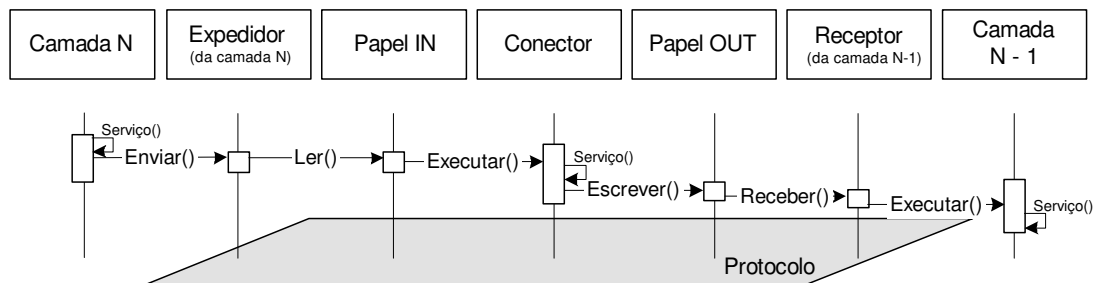
Figura 12: Estrutura dinâmica do estilo camadas
