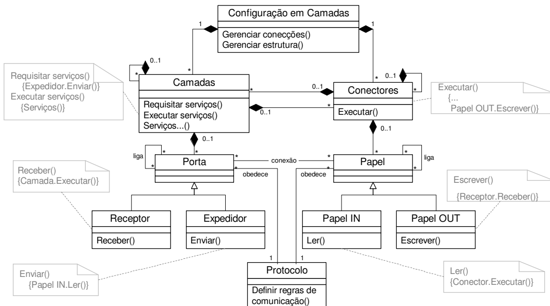
Figura 3: Estrutura estática do estilo camadas
